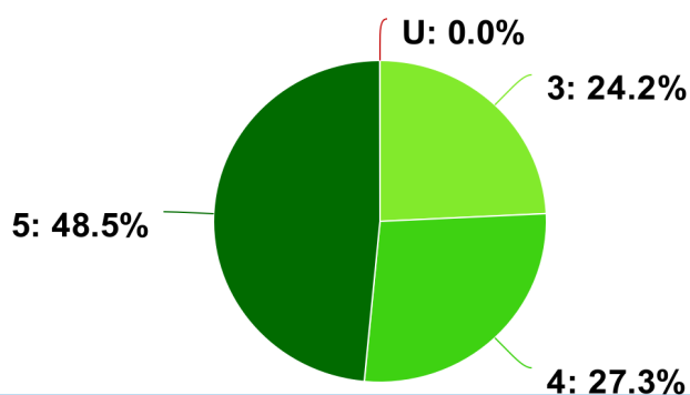
Speciell relativitetsteori [FUF045]
