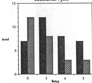
Subatomär Fysik
